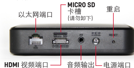
后面板
